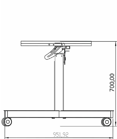
Modalità Tavolo Altezza minima / Configurazione del supporto: 700 mm
