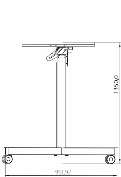
Modalità Tavolo Altezza massima / Configurazione del supporto: 1350 mm
