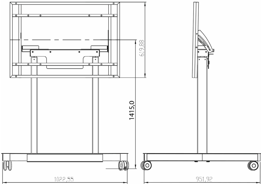
Altezza massima / Configurazione del supporto: 1415 mm
