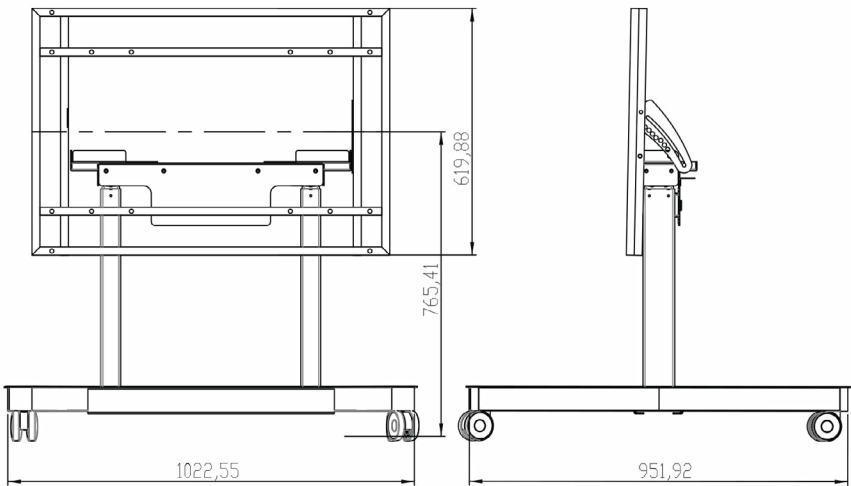
Altezza minima / Configurazione del supporto: 765 mm
