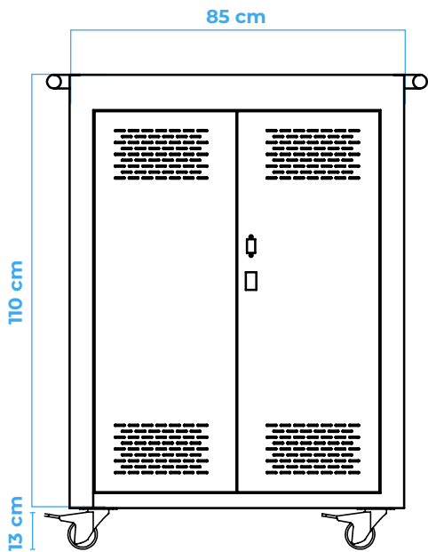
Vista frontale
